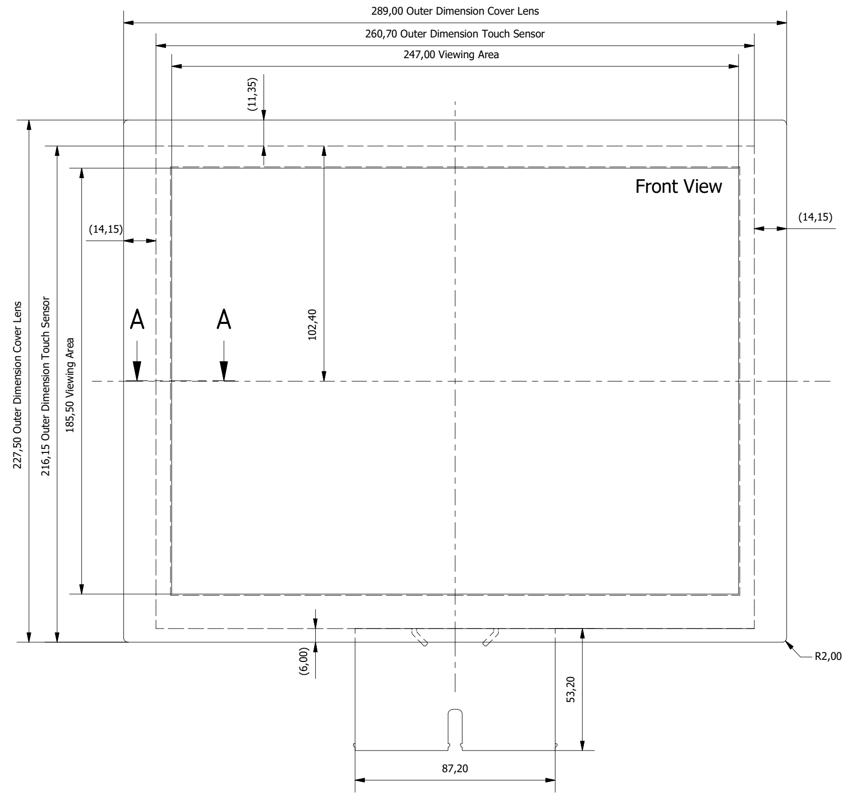
A-A ( 3 : 2 )
