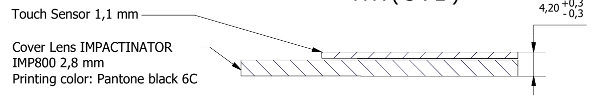
A-A ( 3 : 2 )
